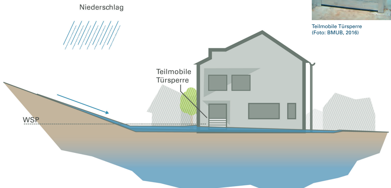
Abbildung 23 Skizze zu möglichen mobilen Türsperren (Ingenieurbüro Reinhard Beck)
